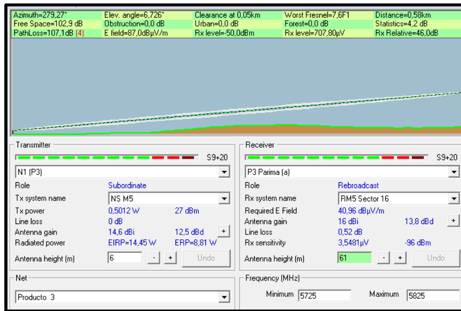
Figura 41: Enlace Nodo 1 – Punto de Acceso Central en Parima (Producto 3) Fuente: Elaborado por las autoras
