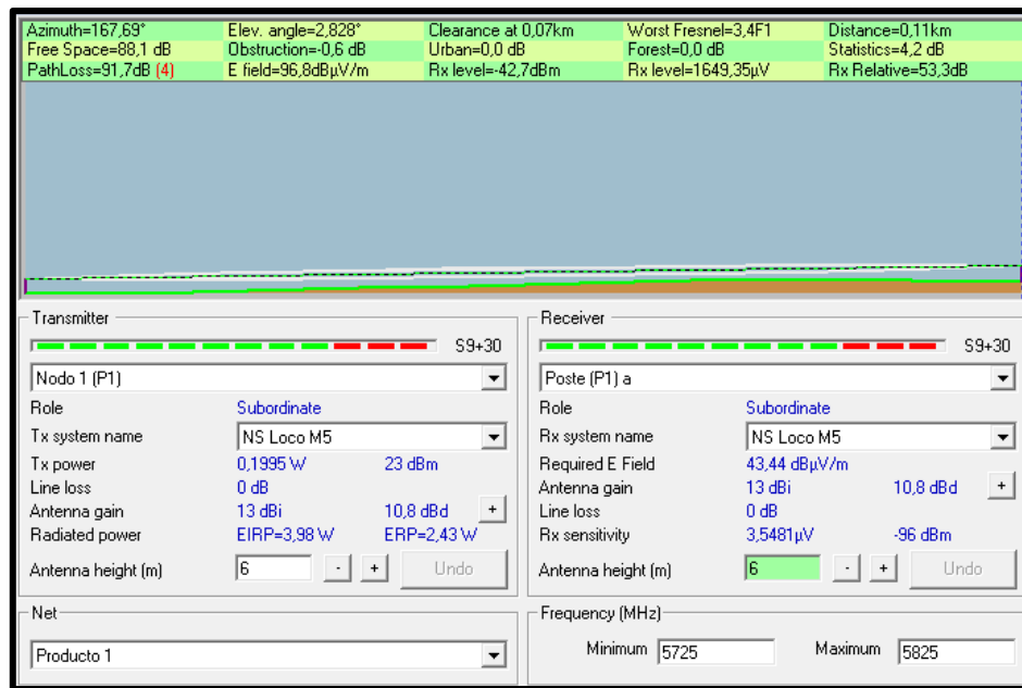
Figura 29: Enlace Nodo 1 - Poste (Producto 1)
