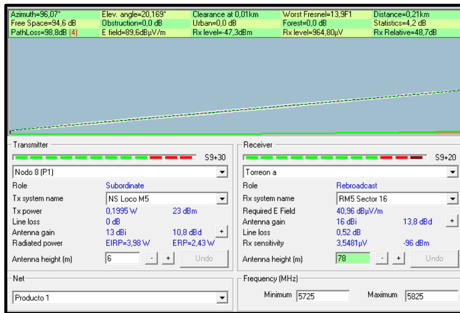
Figura 37: Enlace Nodo 8 - Punto de Acceso Central en Torreón (Producto 1) Fuente: Elaborado por las autoras
