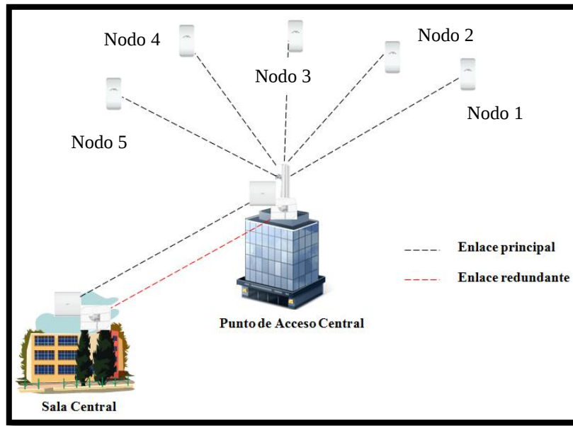
Figura 27: Diseño detallado Producto 3.
