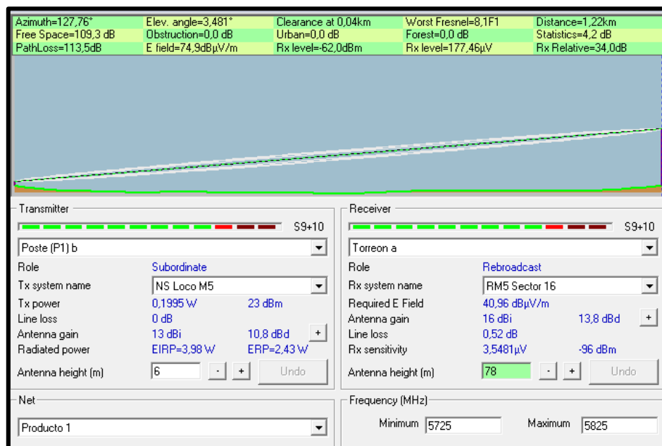
Figura 30: Poste - Punto de Acceso Central en Torreón (Producto 1)
